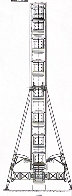
Sezione 1-1 (1:50)
